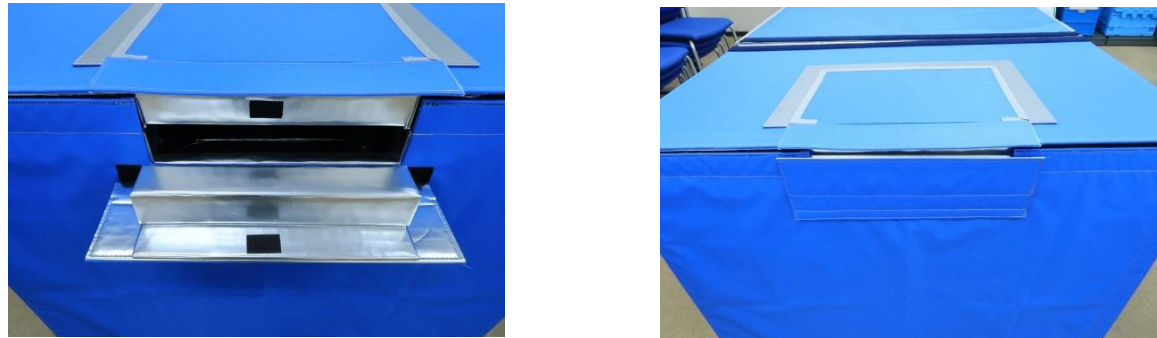
手順9 トップ本体（フロント側）（T1-1）にトップ本体パーツ小（T1-3）を差し込む
