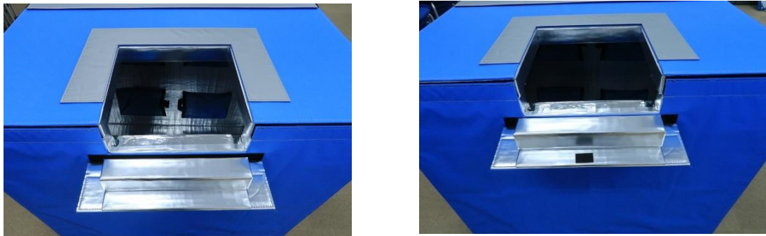
手順7 トップ本体（フロント側）（T1-1）を取付ける
