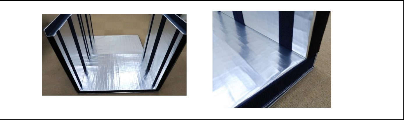
手順3 ボトム(B)にフロント(F)を取付ける
